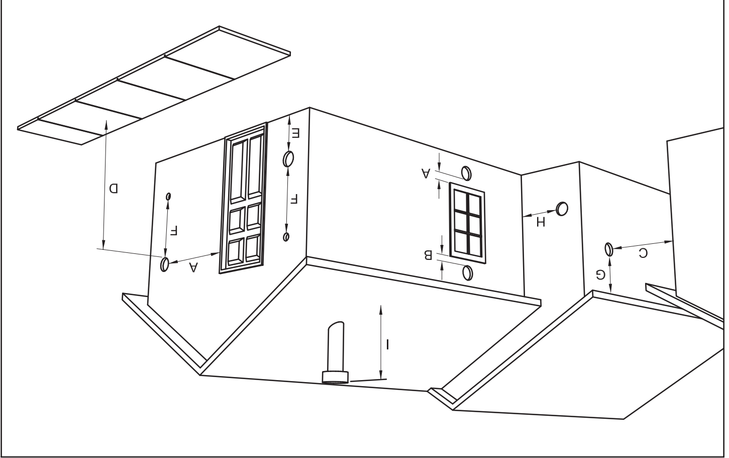
DÉGAGEMENTS POUR LA SORTIE D'ÉVACUATION POUR POËLE À GRANULÉS
