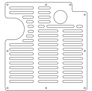
892776 1 Panneau arrière ventilé
