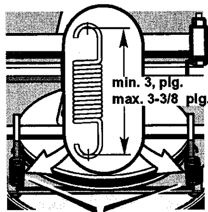
Resorte de propulsión Figura 63
