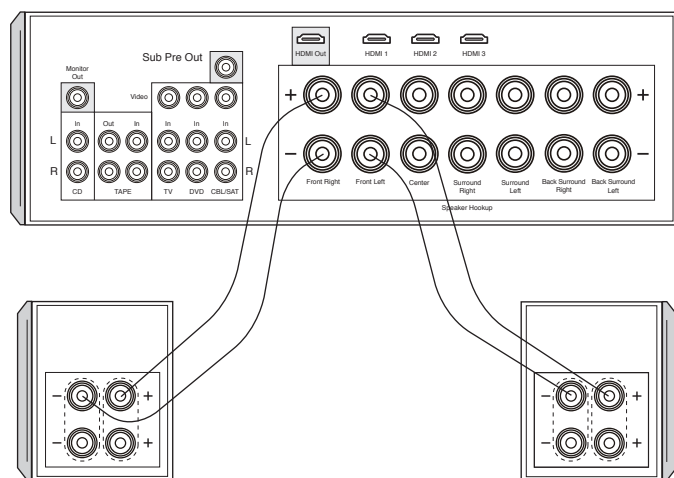
Figura 3 Conexões padrão
