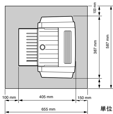
上面図
