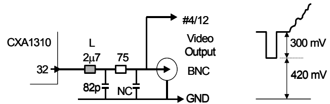
Fig. 4. Video output.
