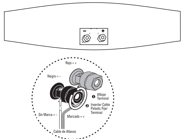
Figura 5. Los altavoces satélite y del canal central presentan terminales que podrán ser conectadas de distinto modos (p.e., a través de conector o cableados directamente, tal como le muestra la imagen).
