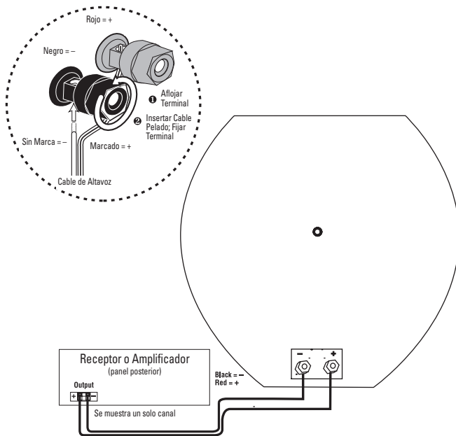
Figura 4. El diagrama de cableado muestra la polaridad de las conexiones de un canal de sistema de cine doméstico.
