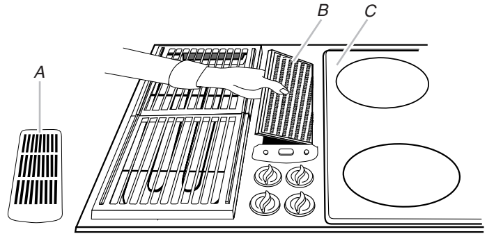
A. Grille de ventilation (précédemment retirée) B. Filtre à graisse amovible C. Module amovible de plaques chauffantes
