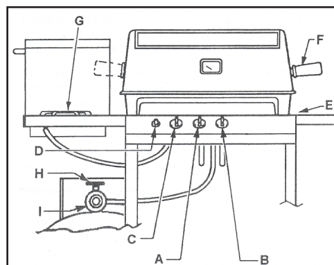
A. BRÛLEUR GAUCHE B. BRÛLEUR DROIT C. BRÛLEUR LATÉRAL D. ALLUMEUR E. ORIFICE D'ALLUMAGE F. POIGNÉE G. BRÛLEUR LATÉRAL H. SOUPE DE LA RÉSERVOIR I. RÉGULATEUR
