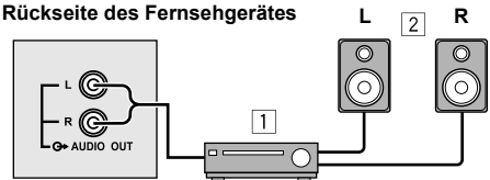
Rückseite des Fernsehgerätes
