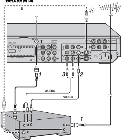
接收器背面
