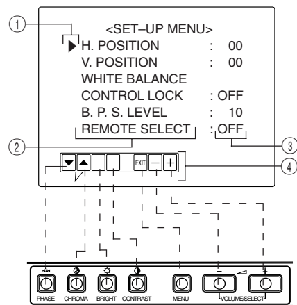
<Botón del panel frontal>
