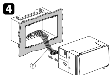
Car dashboard / Cubretablero del automóvil / Tableau de bord de la voiture
