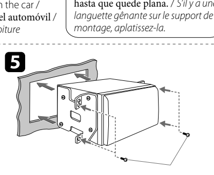
Screw removed from the car / Tornillo removido del automóvil / Vis retiré de la voiture
