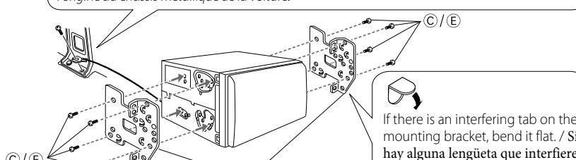
Car dashboard / Cubretablero del automóvil / Tableau de bord de la voiture
