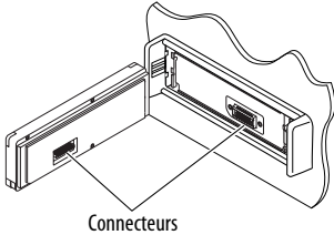
Connecteurs
