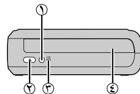
① زر الطاقة (I/O) ② زر الإخراج ③ مؤشر الطاقة ④ حاوية القرص
