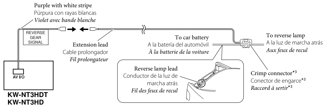
Reverse lamp Luz de marcha atrás Feux de recul
