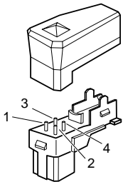
Angebrachte 4 Anschlussfahnen
