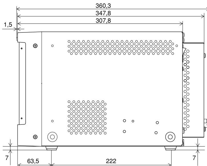
Seitenansicht
