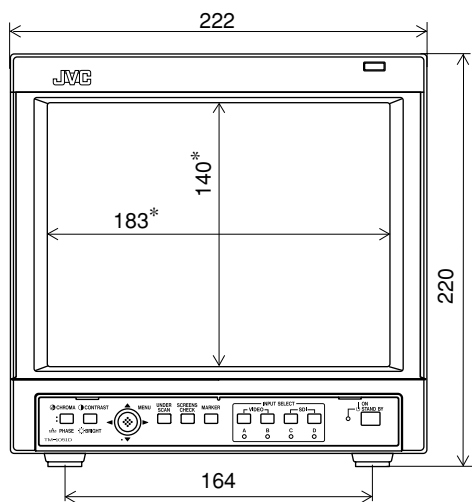
Vorderansicht
