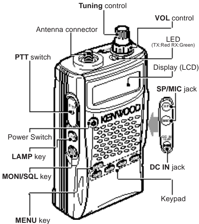
TH-K2E/ K4E
