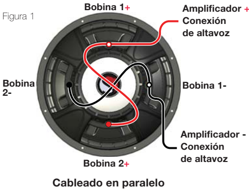
Cableado en paralelo
