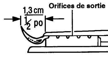
Flamme typique d'un brûleur, à la puissance maximale
