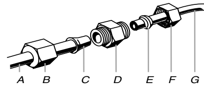
A. Tubería de agua del refrigerador B. Tuerca (provista) C. Bulbo D. Acoplamiento (adquirido) E. Férula (adquirida) F. Tuerca (adquirida) G. Línea de agua de la casa
