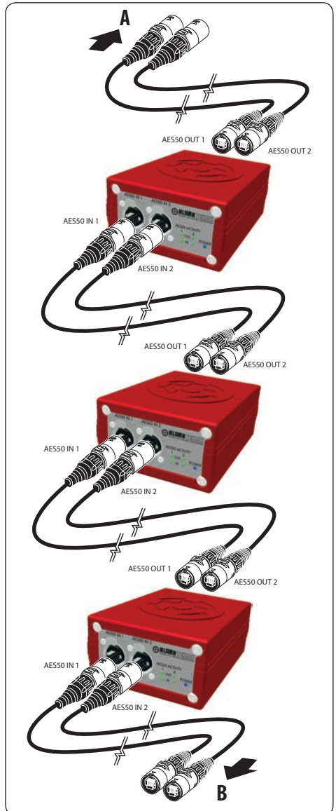
Schéma de connexion typique entre plusieurs boîtiers (par exemple, trois boîtiers connectés en série). A. Vers l'horloge esclave. B. Vers l'horloge maître.
