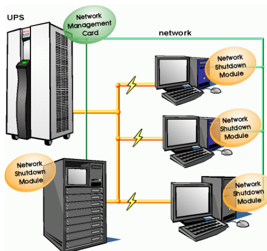
connexion avec Network Management Card
