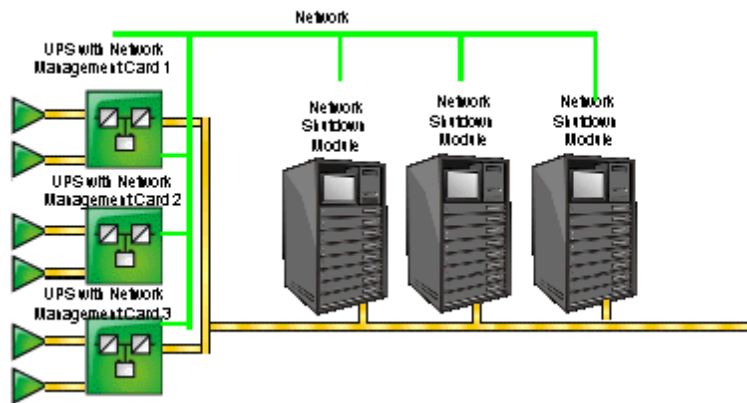
Trois onduleurs en parallèle alimentant plusieurs serveurs
