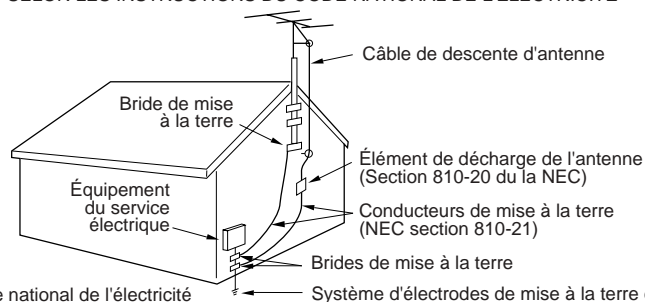
EXEMPLE DE LA MISE À LA TERRE DE L'ANTENNE SELON LES INSTRUCTIONS DU CODE NATIONAL DE L'ÉLECTRICITÉ
