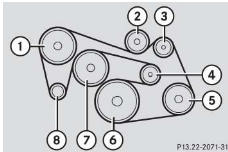
C 230 Kompressor
