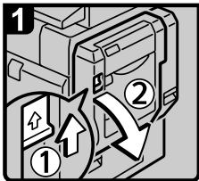
• Open the duplex unit.
