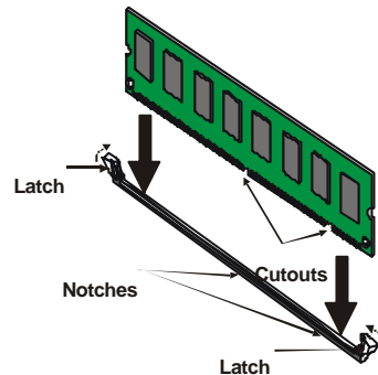
SDRAM Module
