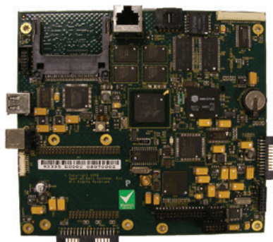
PCB-006
