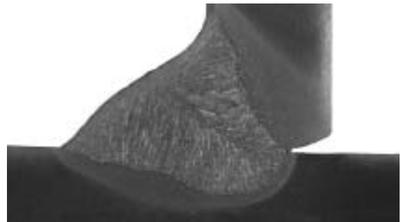
8 mm Horizontal Fillet
