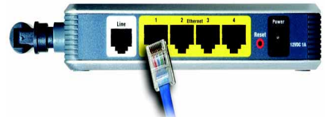
Figura 4-2: Collegamento di un PC
