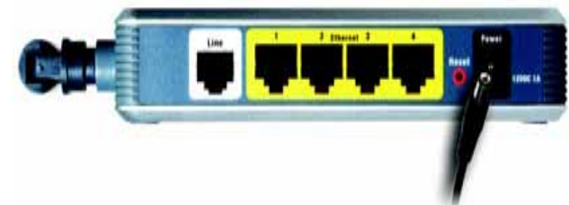
Figura 4-5: Conexión de la alimentación
