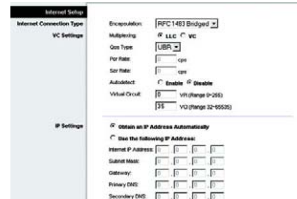
Figure 5-3 : RFC 1483 Bridged - Dynamic IP (RFC 1483 Bridged - Adresse IP dynamique)
