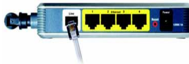
Figura 4-1: Ligar a linha ADSL
