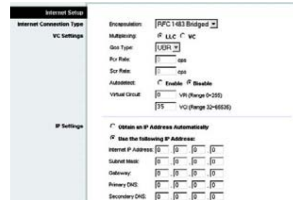
Figure 5-4 : RFC 1483 Bridged - Static IP (RFC 1483 Bridged (ponté) - Adresse IP statique)
