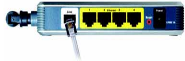
Figura 4-4: Conexión de la línea ADSL
