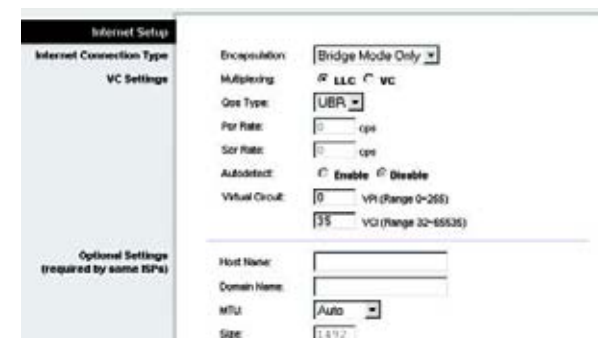
Figur 5-8: Bridged Mode Only (Kun Bridged-tilstand)
