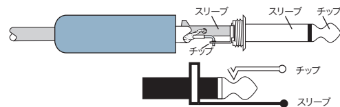
図 C：TS プラグ
