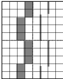
Upper: WF6 Lower: WF1 1DIV: 0.2V 2DIV: 5V 5ms TP1403 ENV.
