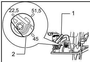
1. Palanca 2. Tope de seguridad
