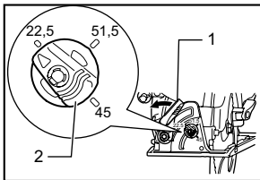
1. Levier 2. Butoir positif
