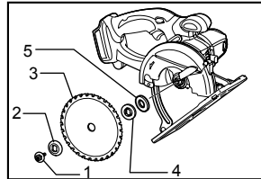
1. Boulon hexagonal 2. Bague externe 3. Lame 4. Flasque intérieur 5. Rondelle à coupelle
