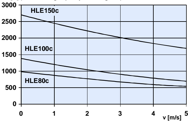
F_y [N]
