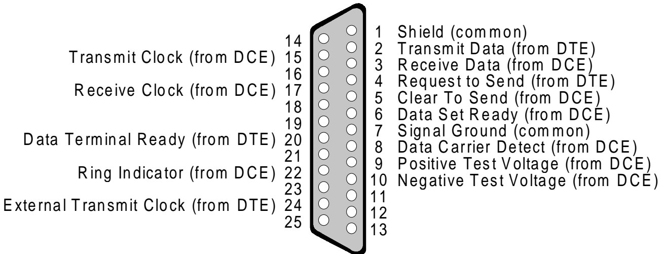
RS-232 Pin Out
