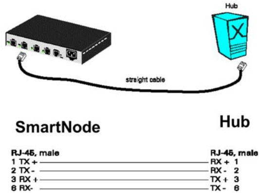
Câble droit
