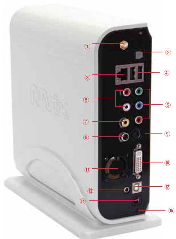
제품 뒷면
