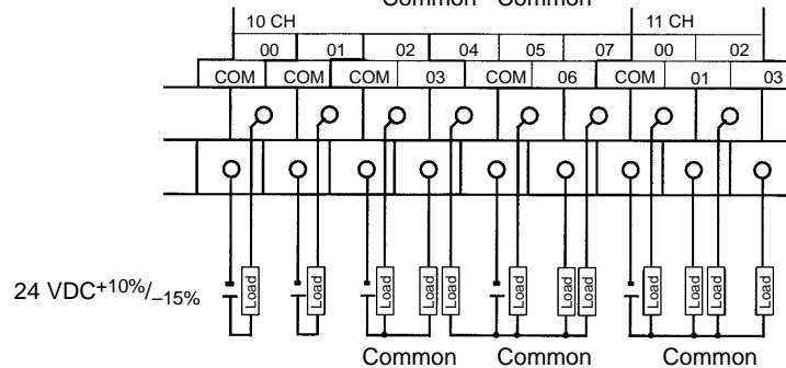
CPM1A-30CDT-D
