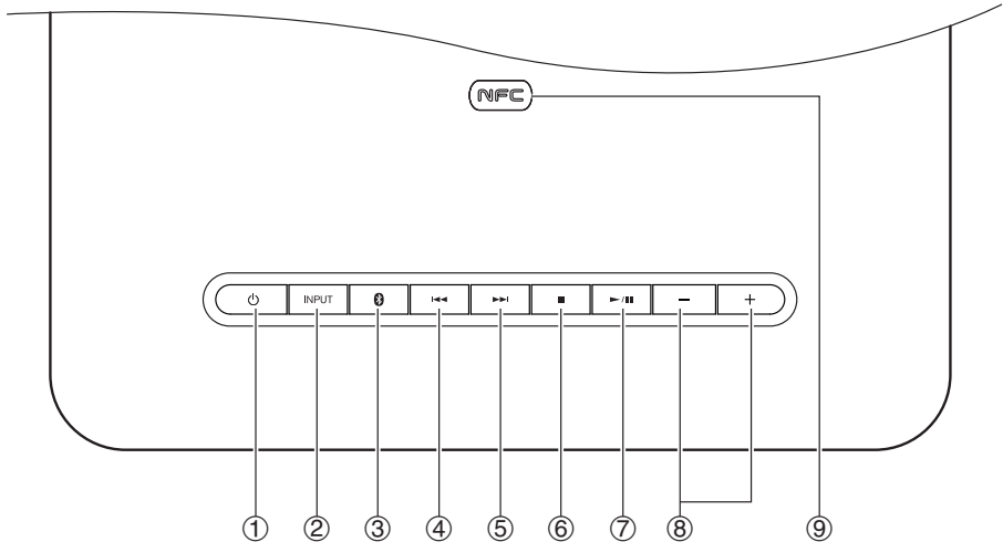
Pannello anteriore
