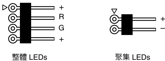
圖 8。 整體與聚集 LED 插腳，EX4650A 與 EX8650A
