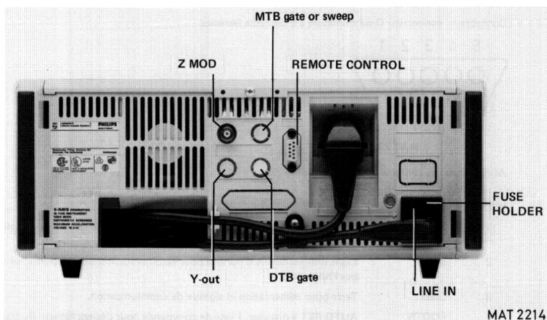
Figure 3.4 Vue arrière de l'oscilloscope.
