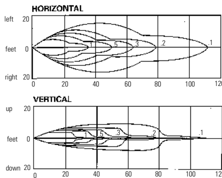
IT18 - 12 Volt, 18 Watt, Tungsten
