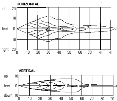
IT12 - 12 Volt, 12 Watt, Tungsten
