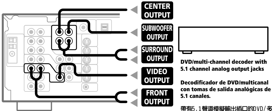
帶有5.1聲道模擬輸出插口的DVD/多聲道解碼器
