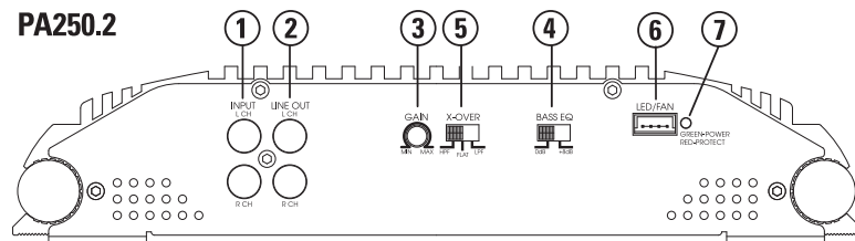
FIGURA 1—CONTROLES Y CONEXIONES DEL AMPLIFICADOR: PANEL DELANTERO (PA250.2)
