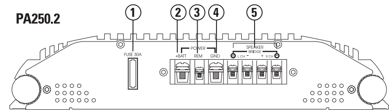
FIGURA 3—CONNESSIONI DELL'AMPLIFICATORE—LATO POSTERIORE (PA250.2)
