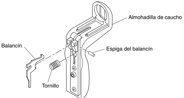
Figura 6 - Retiro del balancín
