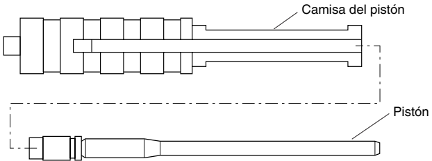
Figura 4 - Retirando el pistón de la camisa
