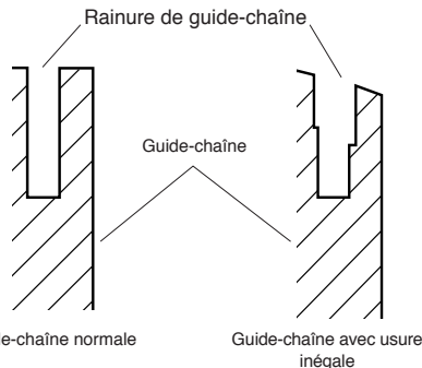
Figure 21- Coupe transversale d'une guide-chaîne montrant une usure inégale
