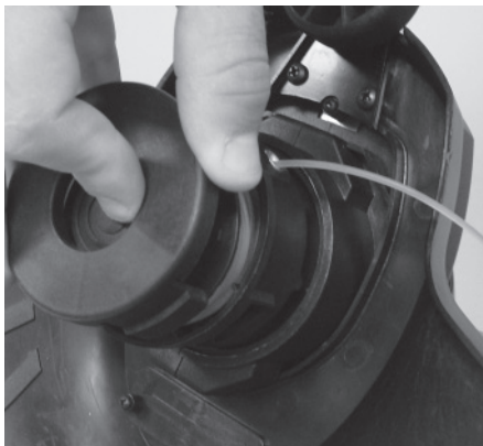
Figura 27 - Reposición del carrete en la carcasa
