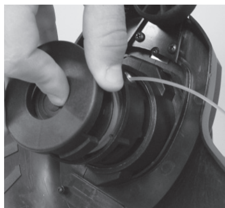
Figure 27 - Mise en place de la bobine dans le boîtier
