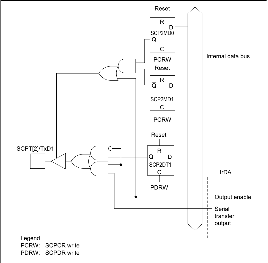
Figure 17.3 SCPT[2]/TxD1 Pin
