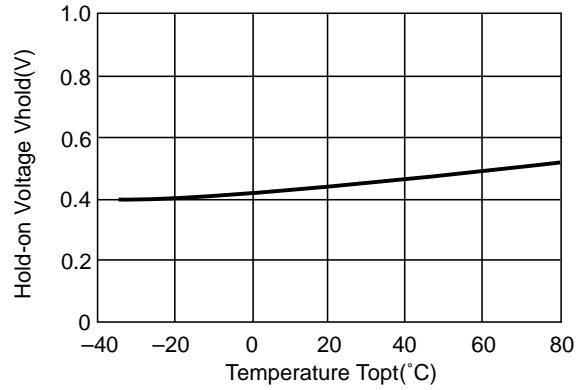
RH5RH501A
