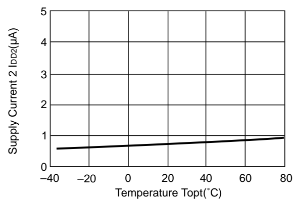
RH5RH501A
